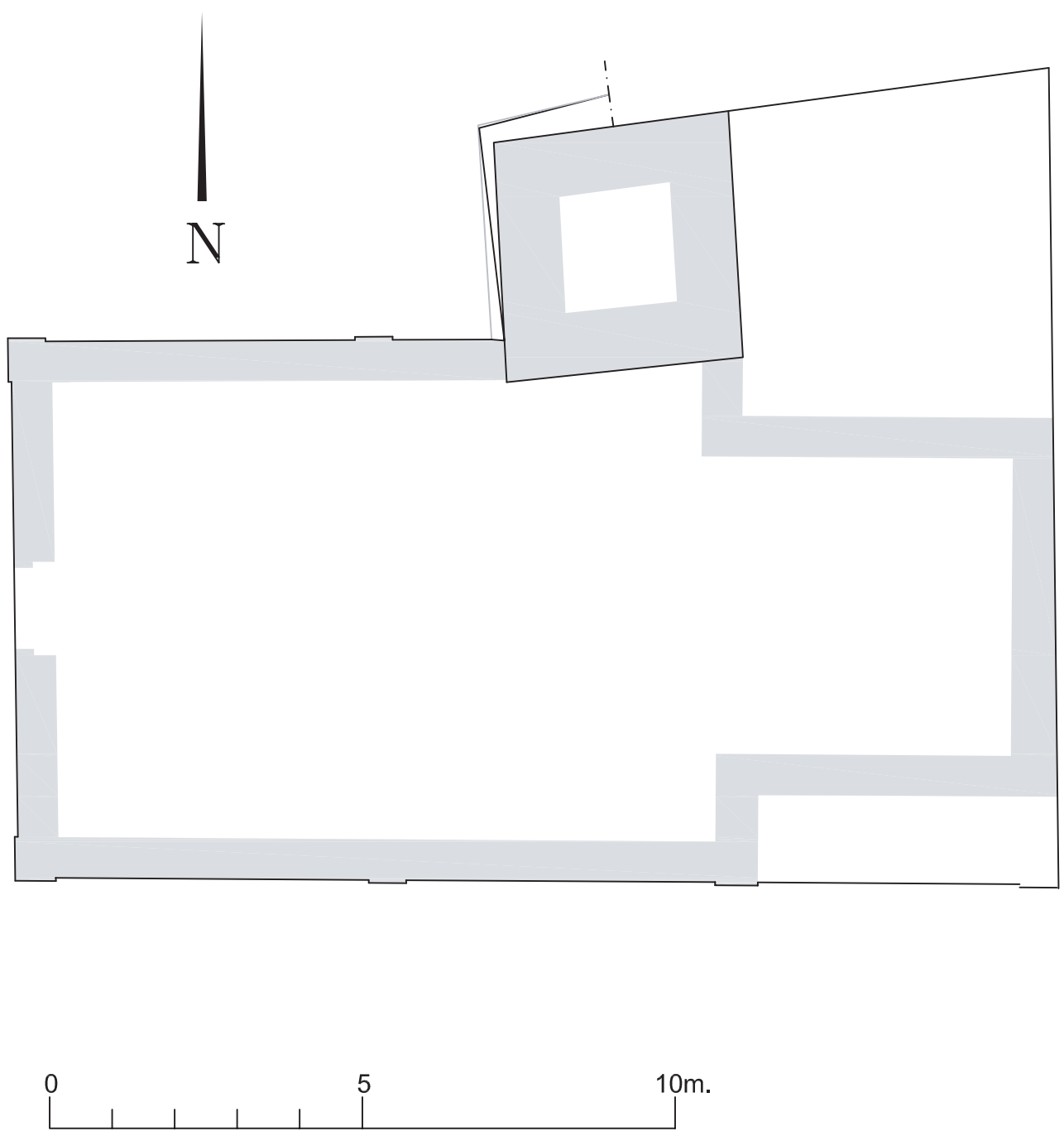
Schematischer Grundriss der Kapelle C.-E. Bettex (Kantonsarchäologie) 6.12.2006
