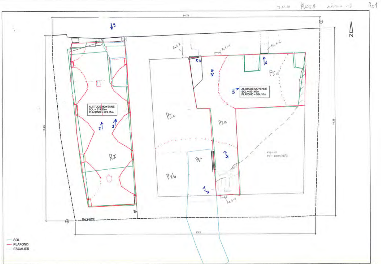
Re1 Sion, Maison Platea. Relevé Géométriques Centre SA, 2014, niveau -2.
