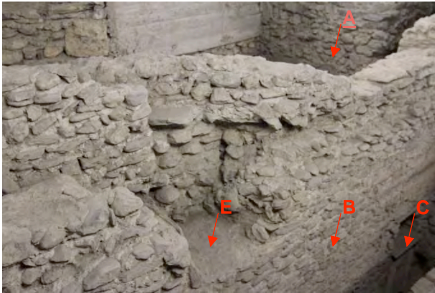
Fig. 3: bassin d'eau froide avec canal d'égouts.
